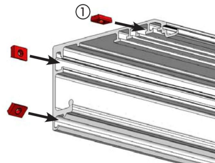
پلیت های پانل های جانبی/ براکت های جانبی
